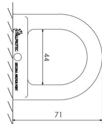
Konfiguracja ścienna
