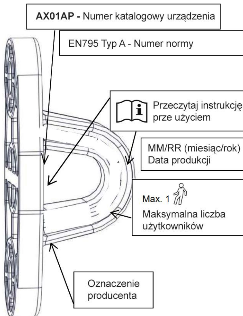
Rys. 3 Sposób oznakowania urządzenia
