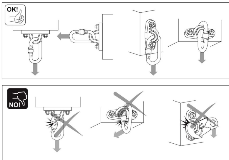
Rys. 12 Podłączanie sprzętu chroniącego przed upadkiem z wysokości do AX01AP
