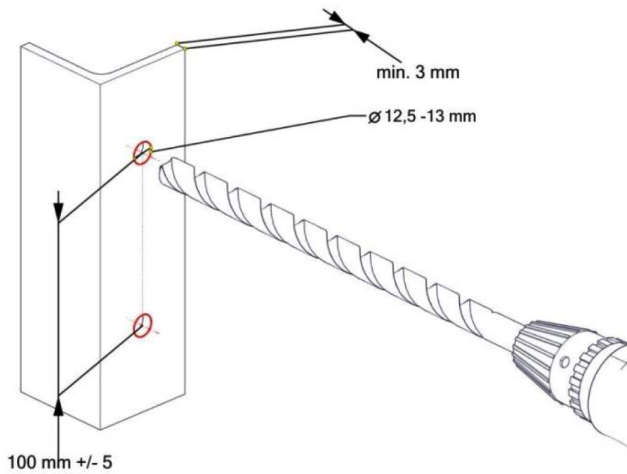
Rys. 4 Wykonanie otworów montażowych w profilach stalowych
