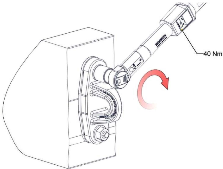
Rys. 11 Dokręcenie kotwy za pomocą klucza dynamometrycznego
