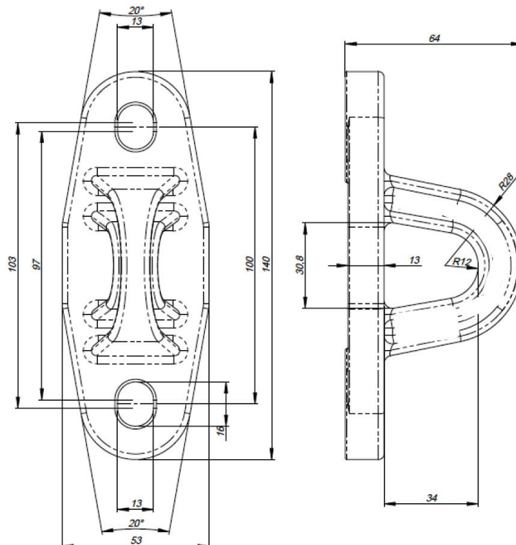
Rys. 2 Wymiary ogólne
