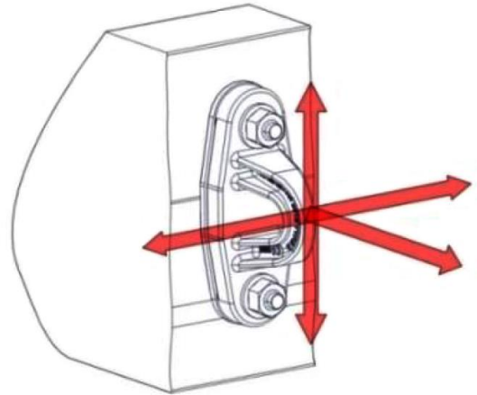
Rys. 1 Dopuszczalne kierunki obciążenia punktu
