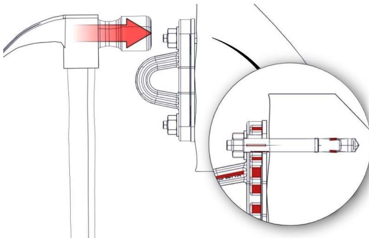
Rys. 10 Osadzanie kotew segmentowych w betonie
