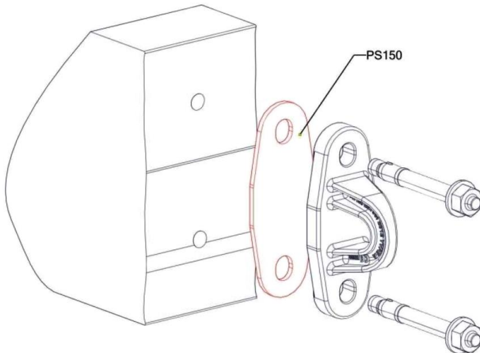
Rys. 8 Umieszczenie podkładki z EPDM pod kotwą
