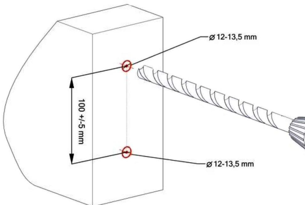
Rys. 9 Wiercenie otworów pod kotwę AX01AP
